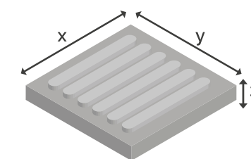
TÁCTIL DE DIRECCIÓN
