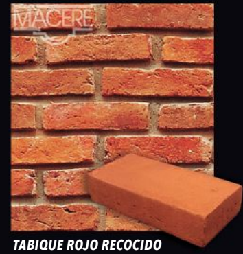
TABIQUE ROJO RECOCIDO • Artesanal • 24 x 12 x 6 cm. aprox. • 58 pzas/m 2 • 1.6 kg/pza.
