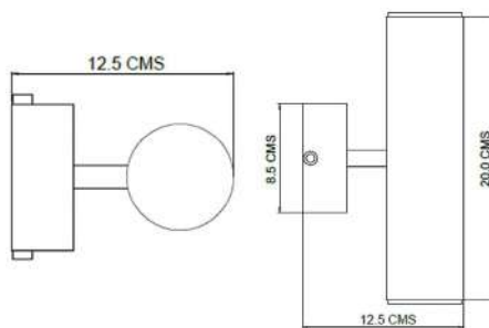
CAD-12-LED-E5-*
