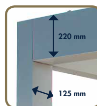
DIMENSIÓN POSTES POLE DIMENSION
