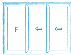
Ventana triple corredizo Ventana fijo - con dos corredizos
