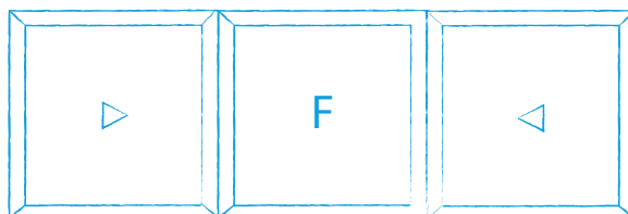
Fijo central y corredizos laterales
