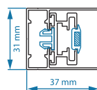
Instalación dentro del hueco
