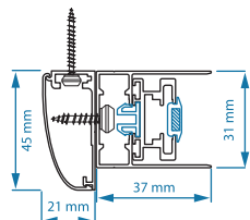
Instalación fuera del hueco
