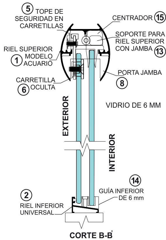
CORTE B'-B' HORIZONTAL
